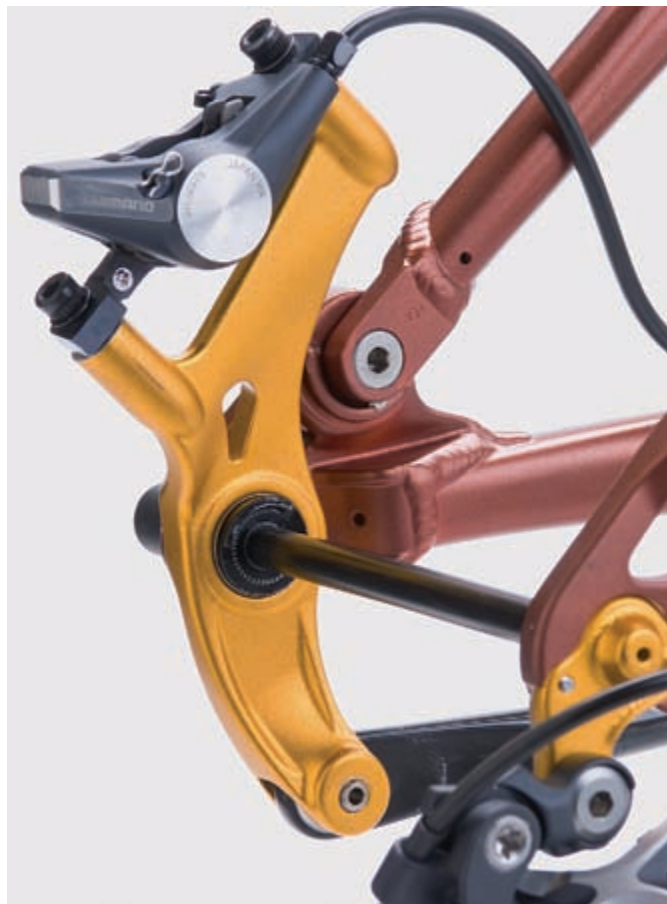
Beim Radausbau verbleibt FLOATING DISC dank ausgeklügelter Befestigung am Ausfallende. Die 10mm Steckachse erhöht die Spursteuigkeit des Hinterbaus und sorgt für eine schleiffreie Disc-Position.
